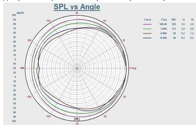
Диаграмма направленности громкоговорителя на разных частотах
